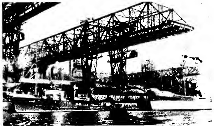
Фрагмент порту металургійного зав. «Озівсталь», обладнаного навантажувально-розвантажувальними механізмами
